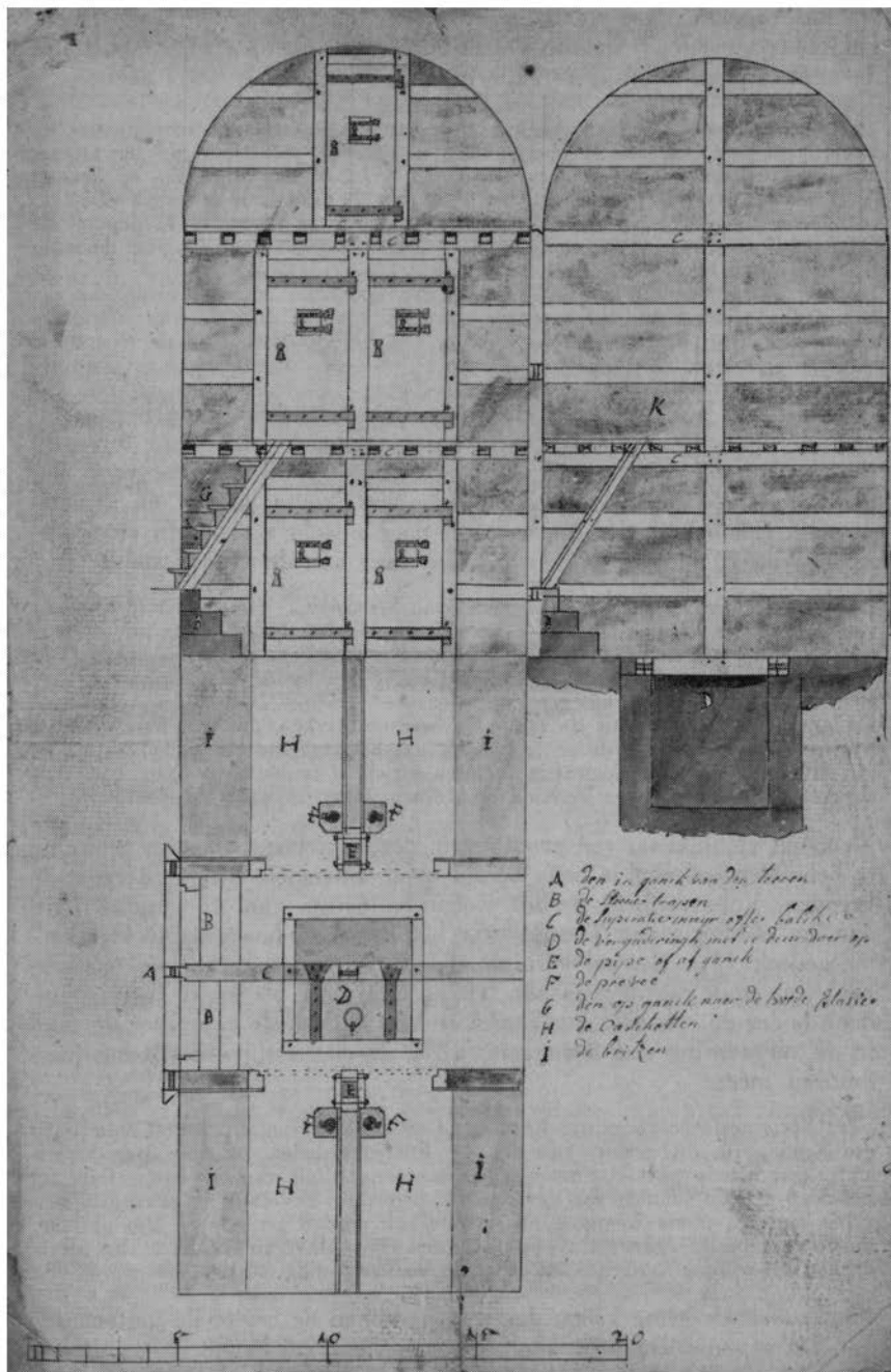
Tekening behorend bij het bestek opgenomen onder voetnota 41) betr. het plan van verbouw anno 1834.
