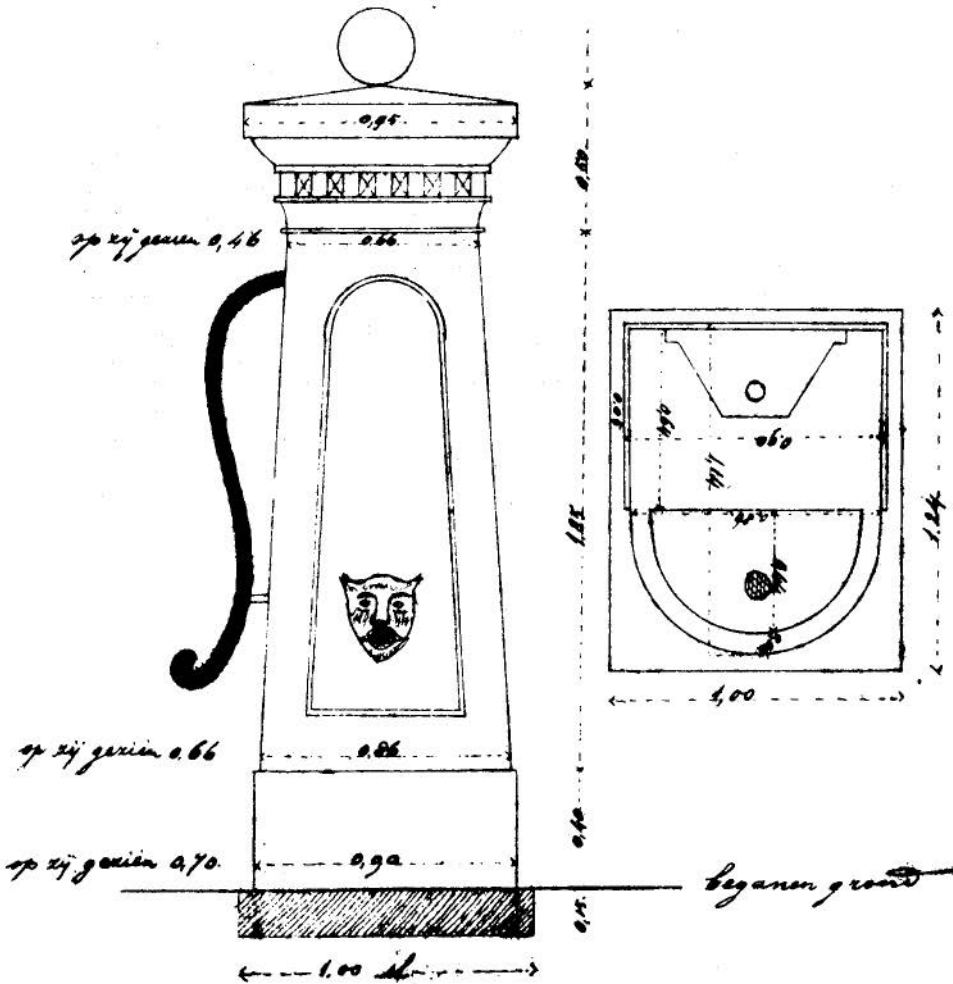
Bestektekening van de pomp op de Veemarkt, 1857.
