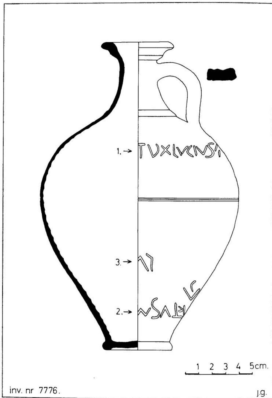
Romeinse kruik van de pottenbakker Lucius uit Coriovallum-Heerlen. Reconstructie en tekening J. K. Gielen.
