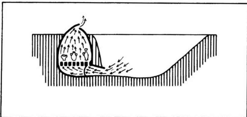
Afb. 1: reconstructietekening van een pottenbakkersoven. (naar A. Bruyn)
