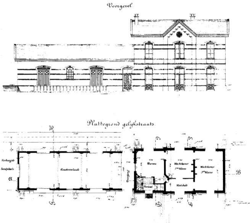
Bestektekening station Heerlen, schaal 1:100 (tot 28% verkleind)
