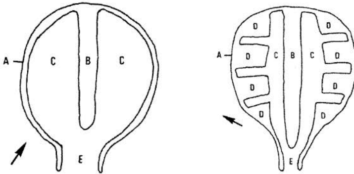
Plattegrond van links de pottenbakkersoven in de Schinkelstraat (1962) en rechts de oven in de Van der Maesenstraat (1996). A oranje-bruin gebrande ovenwand, B middendam, C stook- of heteluchtkanalen, D steunberen, E stookmond.
