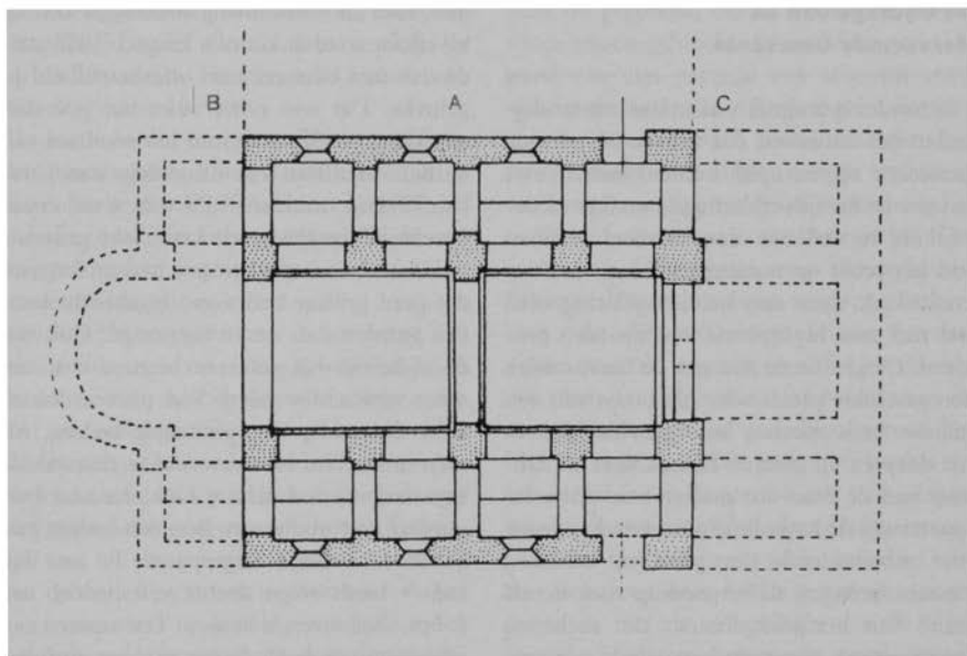
Plattegrond van de Pancratiuskerk in de oudste periode [12de eeuw]. A. Schip. B. Reconstructie koor en absis. C. Reconstructie westbouw
