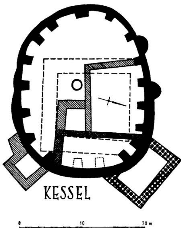
Plattegrond van de ruïne van het motte-kasteel Kessel
