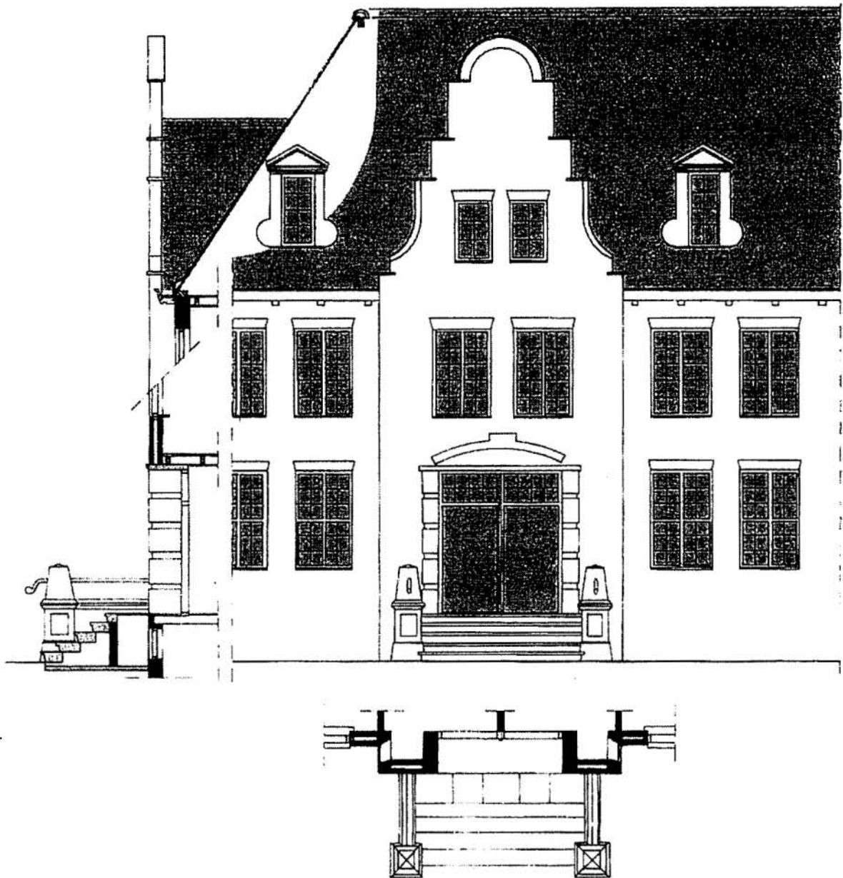
K. Gonser en H.G. Oechler: geveltype RE III in de 'Hermann Goeringkolonie'. [Reconstructietekening H. van der Zanden].
