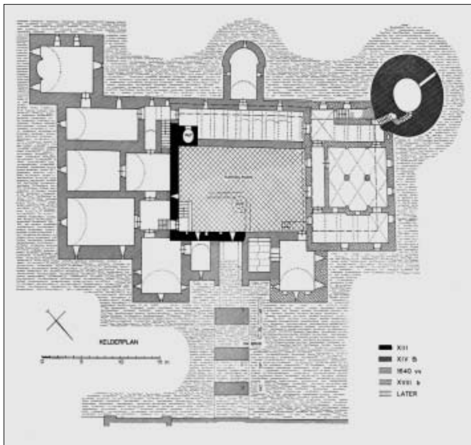
Plattegrond van de kelders van het kasteel op basis van de verkenningen door G. Wisse van de Rijksdienst voor de Monumentenzorg bij de restauratie en in 1954. De weergegeven faseringen en details vormen de basis voor de reconstructietekeningen. Aan de westzijde is een keienvloer aangetroffen. Hier zal zich dus het binnenplein hebben bevonden. Aan de oostzijde is een tussenmuur en een waterput zichtbaar. Tevens zijn in de noord- en oostmuur schiet- of ventilatiesleuven en nissen aangetroffen. Ook zijn er sporen van gewelven waargenomen. Hier heeft zich dus het woongebouw bevonden. De plaats van de tussenmuur geeft de karakteristieke onderverdeling van het woongebouw weer in een derde en tweede deel.
