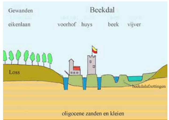
Figuur 4: Model voor vestiging van een kasteel in een beekdallandschap
