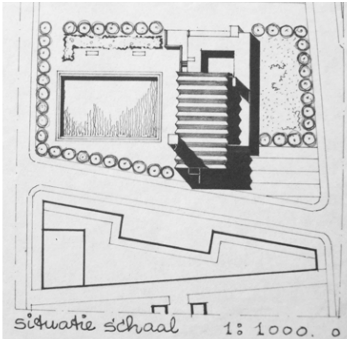
Schetsontwerp kerk 8 en pastorie 9 .
