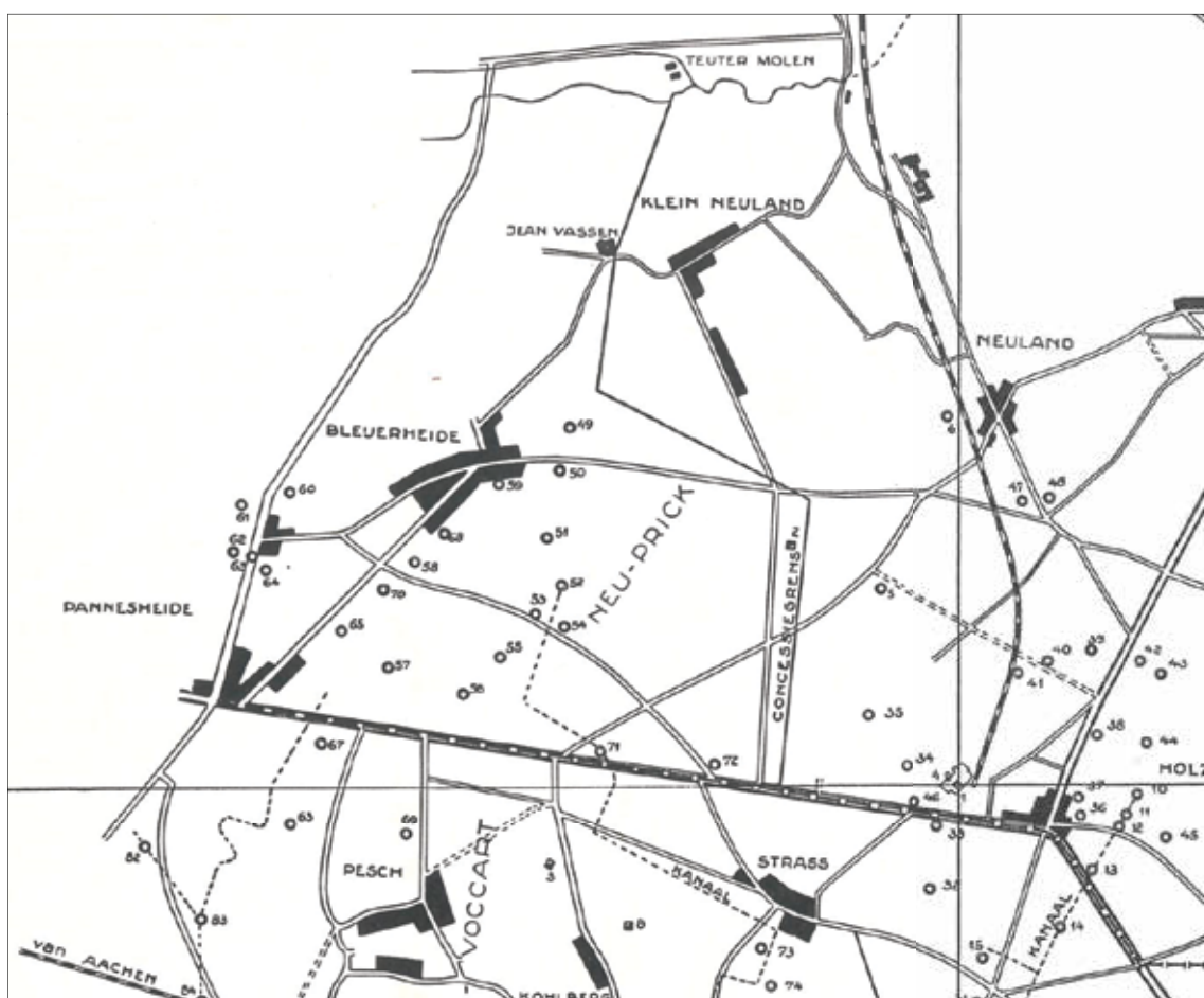
Afbeelding 2 - Situatieplan van de oude schachten in het veld van de Domaniale Mijn en buurmijnen. In: A.H.W. Martens, Administration des mines, van 1810 tot 1960 : Staatstoezicht op de mijnen. Bijlage bij: Verslag van de inspecteur-generaal der mijnen, 1959 ('s-Gravenhage 1961) (Gedraaid 270 graden. Uitsnede. Holz, Nuland en Bleijerheide)
