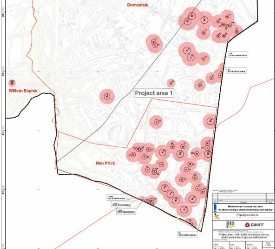
Afbeelding 1 - Project area 1 with shafts of historical mining and impact areas at ground surface level. In: Na-ijlende gevolgen steenkolenwinning Zuid-Limburg (2016) (Uitsnede Holz, Nuland en Bleijerheide)
